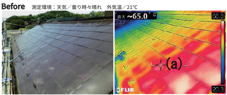
ガイナ塗装前と塗装後の表面温度をサーモグラフィカメラにて比較
